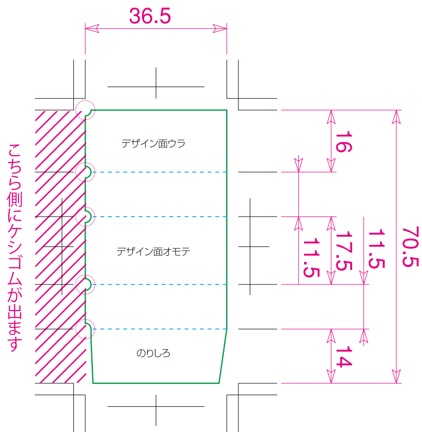
EP-SR-70 長 R 付 (36.5mm×70.5mm)
